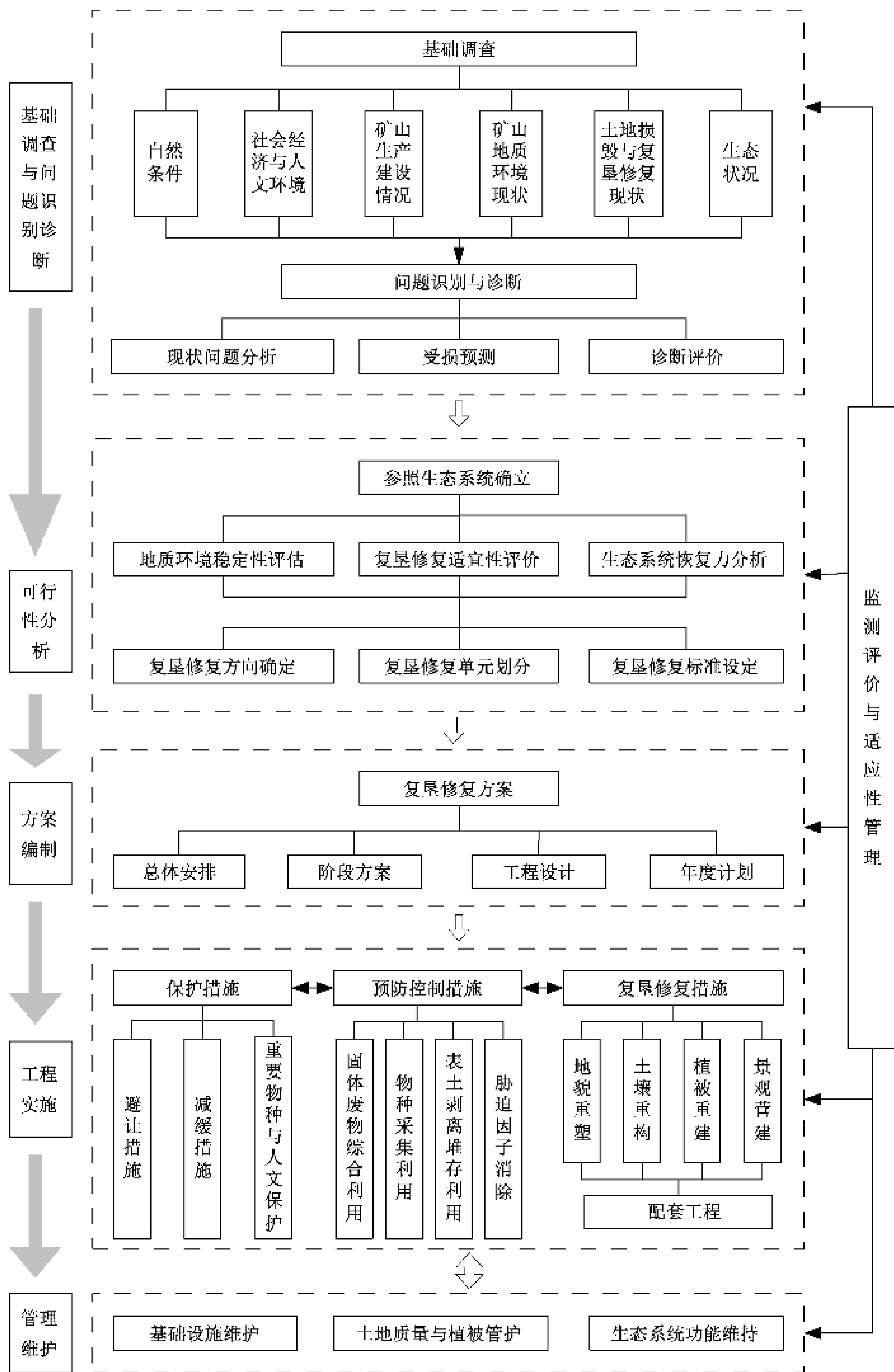
图 1 金属矿复垦修复技术路径
