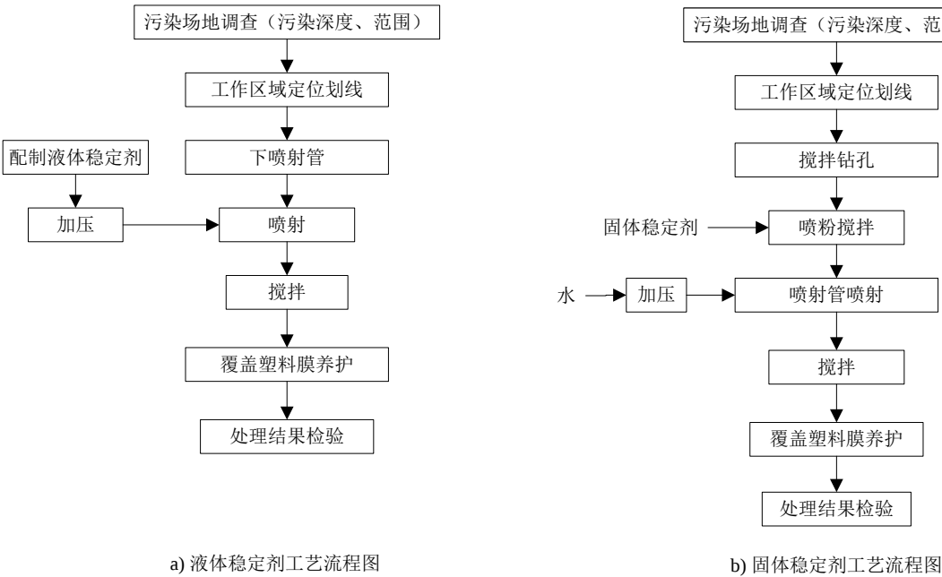
图2 稳定化修复法工艺流程图
