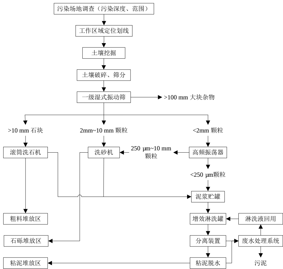
图1 化学淋洗修复法工艺流程图
